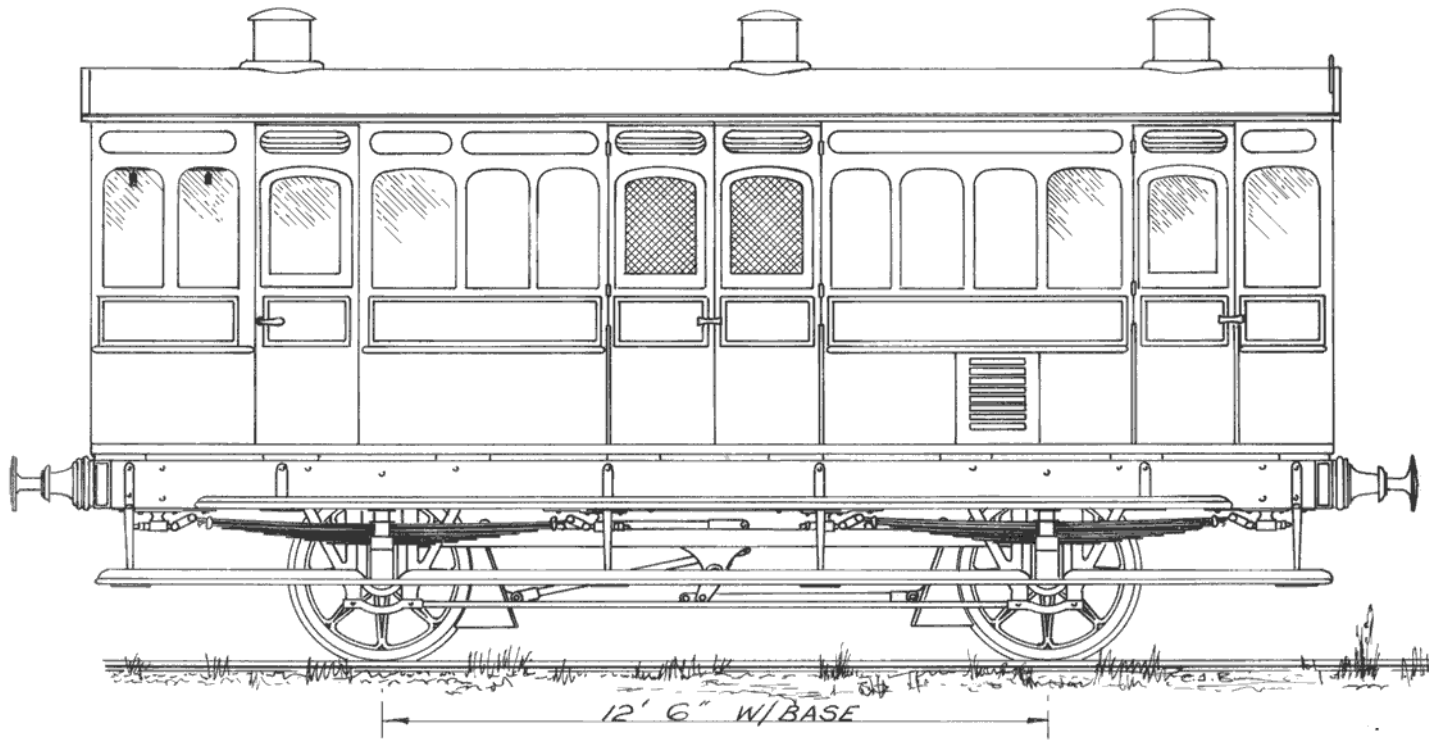
BRAKE VAN. ~
